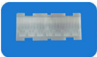
型号：8702-2 焦距：23 角度：125° 距离：15m 尺寸：44*104
